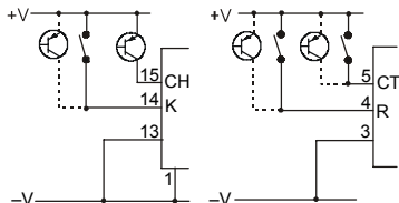
Sourceeingänge (PNP)
