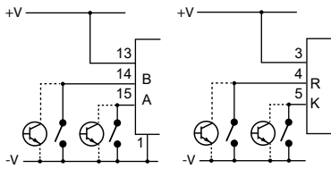
Ingressi Sink (NPN)
